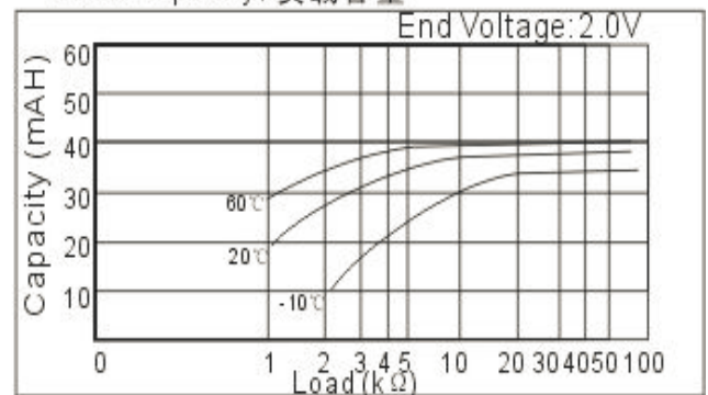
Load-Capacity / 负载容量
